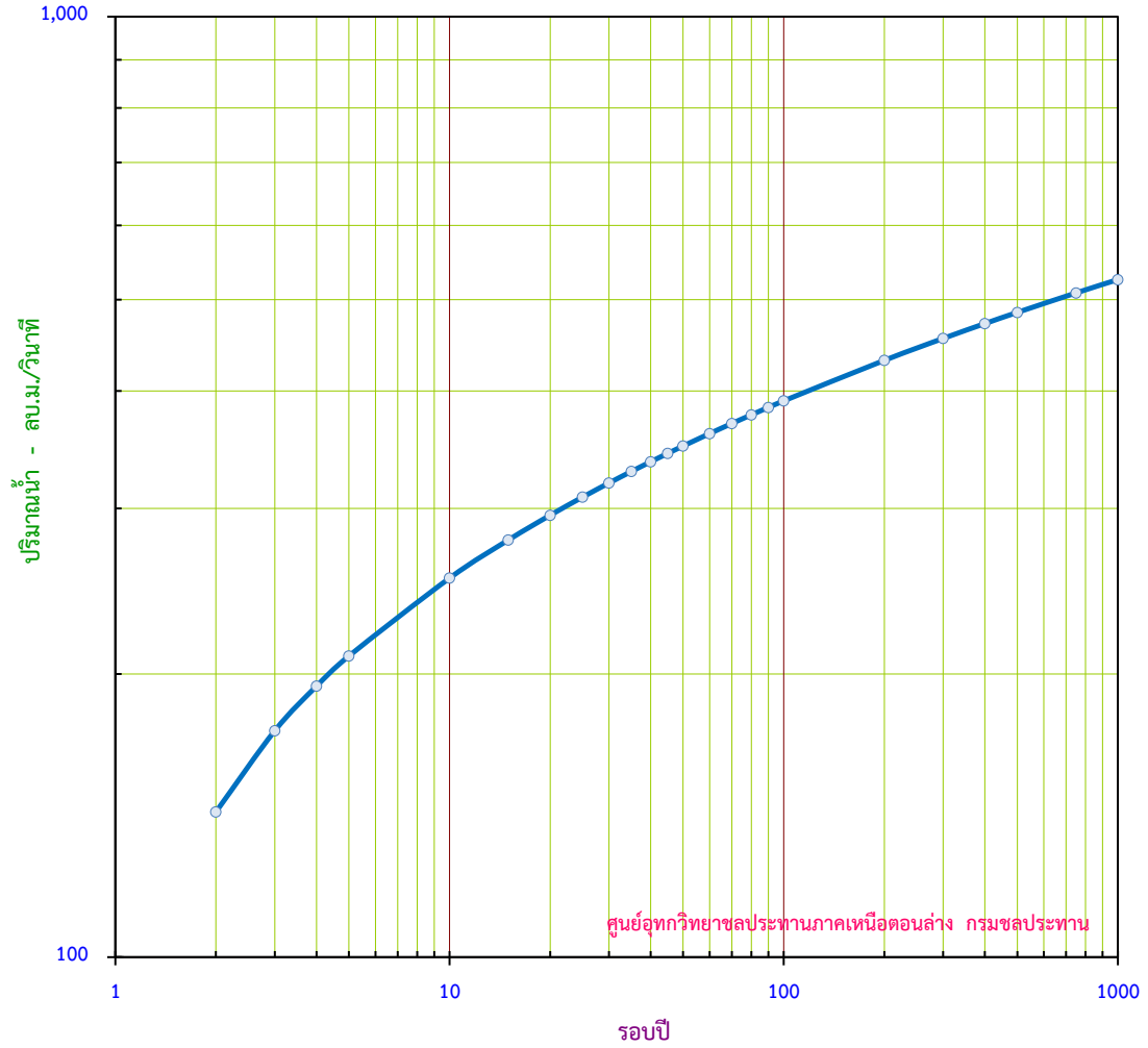
กราฟแสดง ปริมาณน้ำสูงสุดรายปี ขนาดรอบปีต่างๆ สถานี S.3 อ.ห่มสั๊ก จ.เพชรบูรณ์
